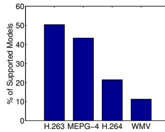
Fig. 3. Video Codecs
