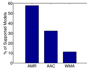
Fig. 2. Audio Codecs
